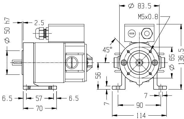
FLANGIA B3-B14/56
